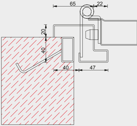
Telaio per combinato
