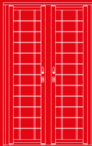
Mod. 2 - Tubo diam 27 mm orizzontale - Piatto orizzontale 30x8
