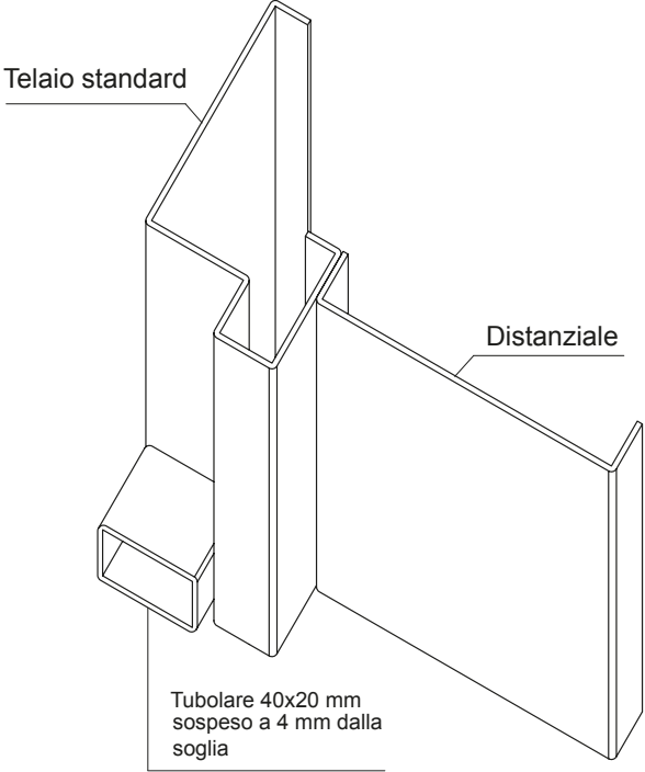
Telaio standard con distanziale da 80 - 100 - 120 mm per grate, persiane e scuroni apribili
