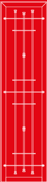
Mod. 1 - tondo diam. 14 - piatto 30x8
