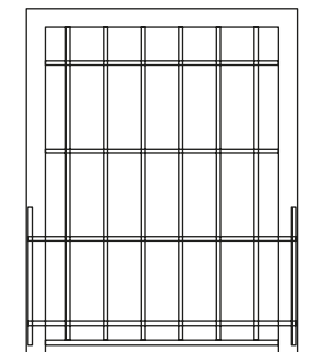
Mod. 7 piatto 40x8 orizzontale e tondo diam. 16 mm verticale
