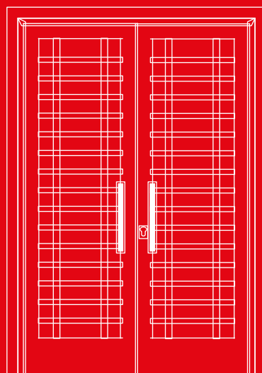
Mod. B - Piatto 25 mm orizzontale - Tondo 12 mm verticale all'interno del vetro camera
