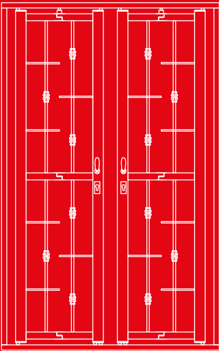
Mod. A - Tondino diam. 14 verticale - Piatto orizzontale 30x8
