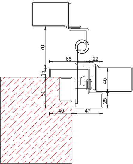
Telaio con cerniera a collo alto
