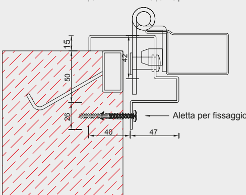
Telaio standard con fori supplementari di fissaggio per persiane, grate e scuroni apribili
