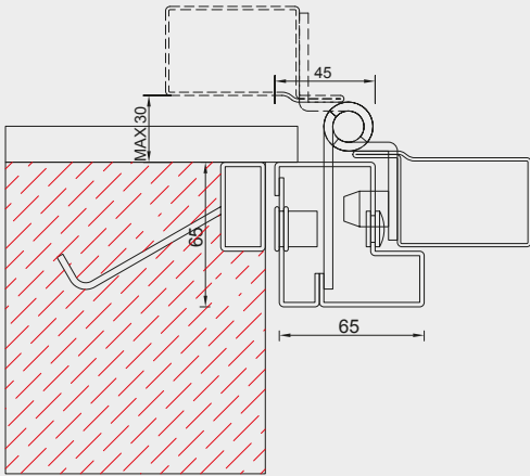
Telaio per persiane modello Onda
