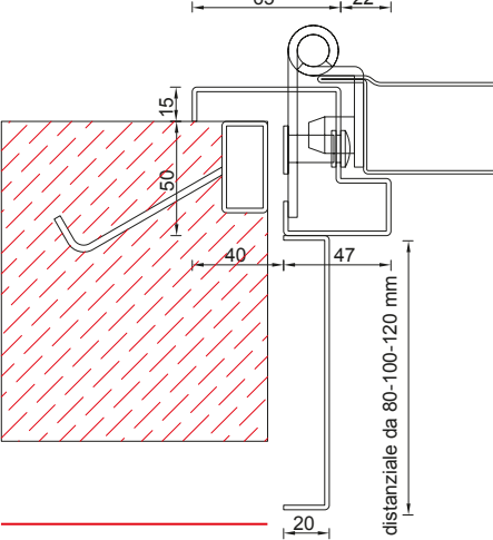
Telaio standard con distanziale da 80 - 100 - 120 mm per grate, persiane e scuroni apribili
