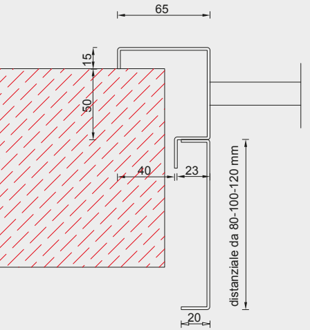
Telaio standard con distanziale da 80 - 100 - 120 mm grate fisse
