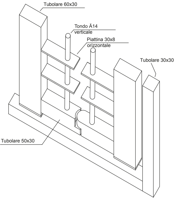
Particolare della grata a snodo
