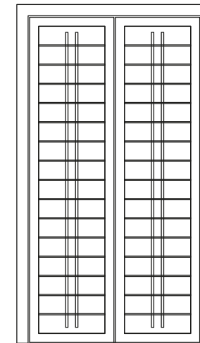
Mod. 7 piatto 40x8 orizzontale e tondo diam. 16 mm verticale
